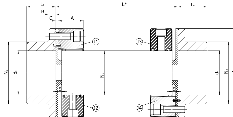
Type GZ
